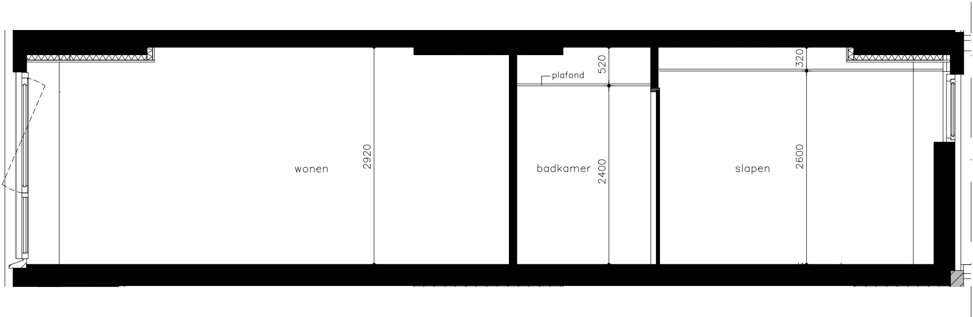
Doorsnede
